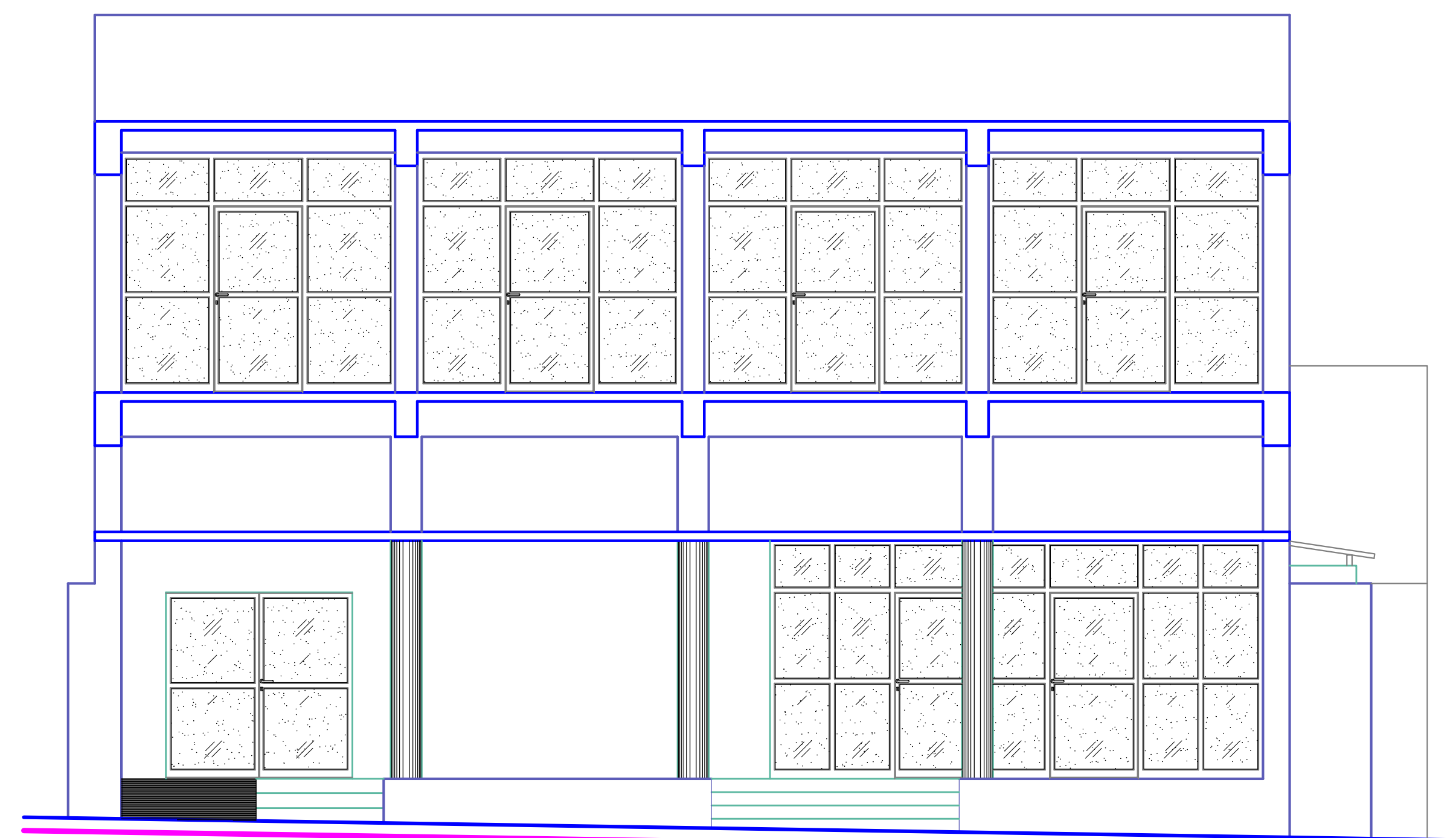
FACHADA ESC. 1:50
